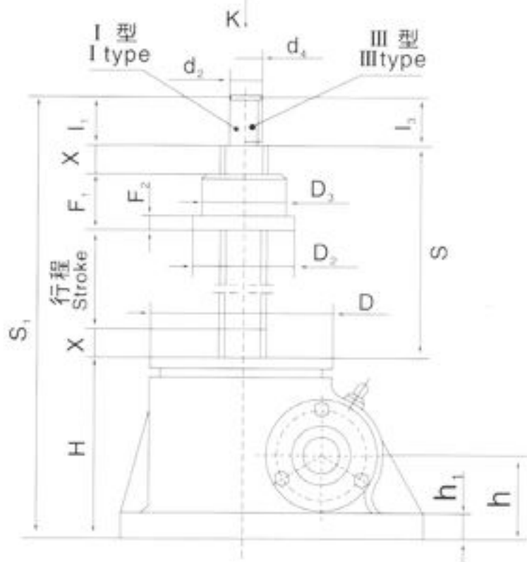
装配型式 A Assembly type A
