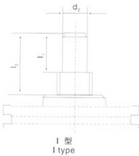
螺杆头部型式 Screw head form
