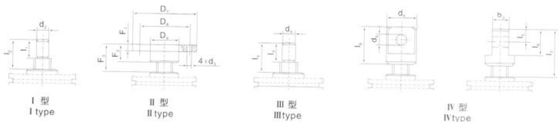
图1 1型结构形式 1 type configuration type
